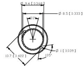
SHAFT MILLING DETAIL 24 TEEHT 2:1
