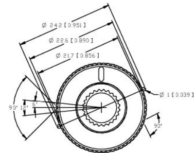
BODY MILLING DETAIL 60 TEEHT 2:1
